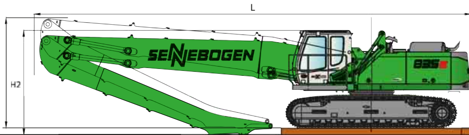
T41/380 tipi alt makine donanımlı 835 R için taşıma ölçüsü
