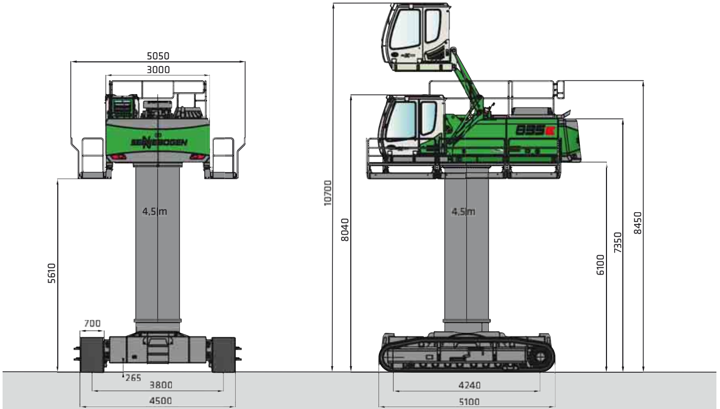
R44D/380 tipi geniş izli alt makine, 4,5 m pilon ve E270 tipi hidrolik olarak yukarı sürülebilir kabin donanımlı 835 R
